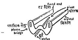
स्टीरियो पिकअप में क्रिस्टलों का जोड़ा । मुर्दा की गति एक प्लास्टिक सेतु द्वारा प्रेषित की जाती है ।
