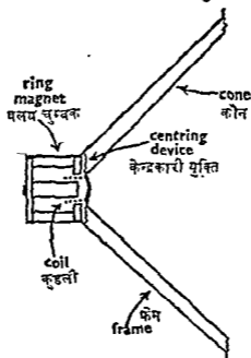
लाउडस्पीकर का संयुक्त: दृश्य ।
