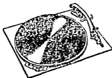
गोल्डरिंग-लेको प्रत्यंजन घूर्णक स्थल और पिकअप।
