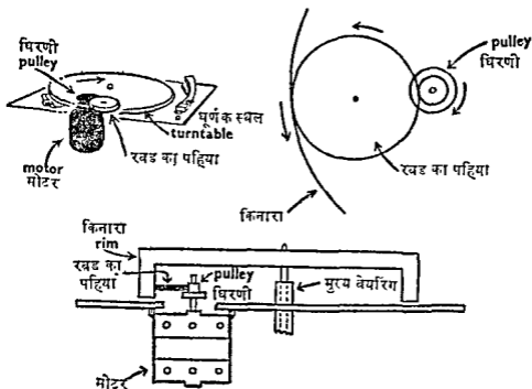
किनारे से घुमाए जाने वाले घूर्णक स्थल के मुख्य भाग।
