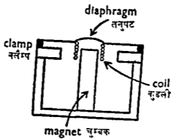
घल-कुंडली माइक्रोफोन का एक रेखाचित्र ।
